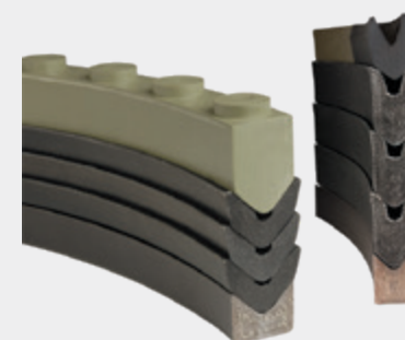
NBR/PLATNO ZAPTIVNI SETOVI VELIKIH PREČNIKA - CARCO TEX
