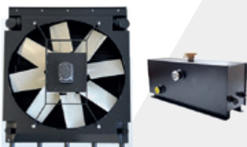
HCC - HLADNJAK ZA DIZEL I GASNE MOTORE sa AC motorom i pumpom Rashladna snaga 1-100 kW Dostupan i sa eksternom jedinicom pampa sa motorom.
