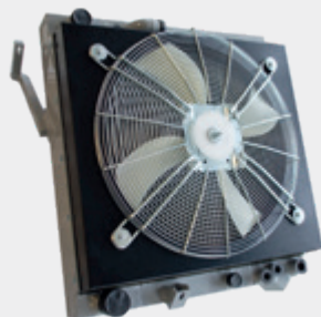
HCC - HLADNJAK ZA DIZEL I GASNE MOTORE Dostupan veliki broj dodatne opreme: Dodatni rezervoari, upravljački sistem za ventilator, spojica za visco ventilator
