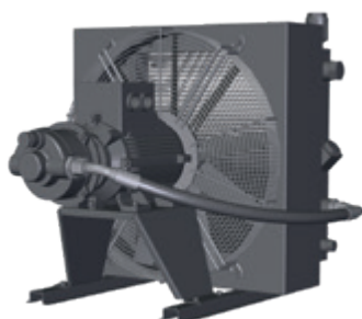
HCP - VAZDUŠNI HLADNJAK sa AC motorom i pumpom Rashladna snaga 1-100 kW Dostupan i sa eksternom jedinicom pampa sa motorom.
