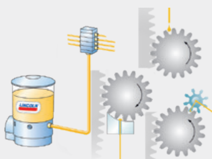
PODMAZIVANJE OTVORENIH ZUPČASTIH PRENOSNIKA
