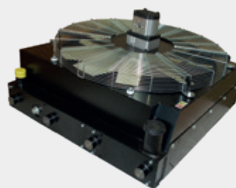
HCC - HLADNJAK ZA DIZEL I GASNE MOTORE Dostupan veliki broj dodatne opreme: zaštita od prašine i kamenja, bajpas cevi ili creva, vazdušna creva...
