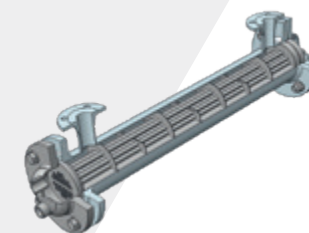
HCT - CEVASTI IZMENJIVAČI TOPLOTE - POPREČNI PRESEK Standardne dužine su do 3m, a prečnici 75-500mm. Postoji mogućnost izrade fiksnih cevi ili cevi koje se vade.
