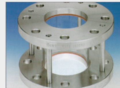
ARMATURA ZA NADZOR PROTOKA
