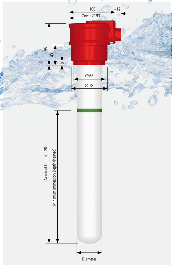
Immersion Heater ROTKAPPE
