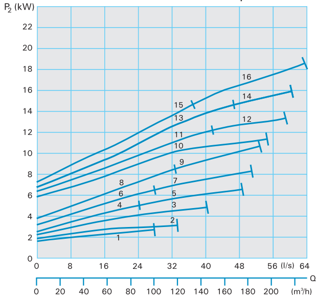
Motor output
